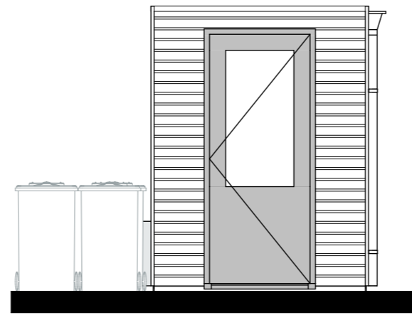
Gevel - tuinzijde
