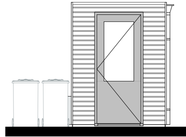
Gevel - tuinzijde (1)
