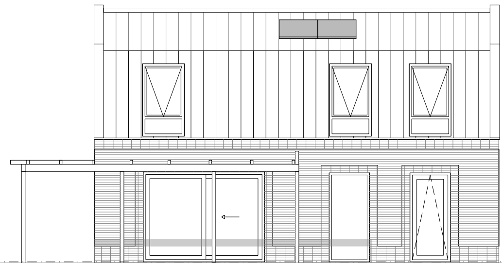
Linker zijgevel
