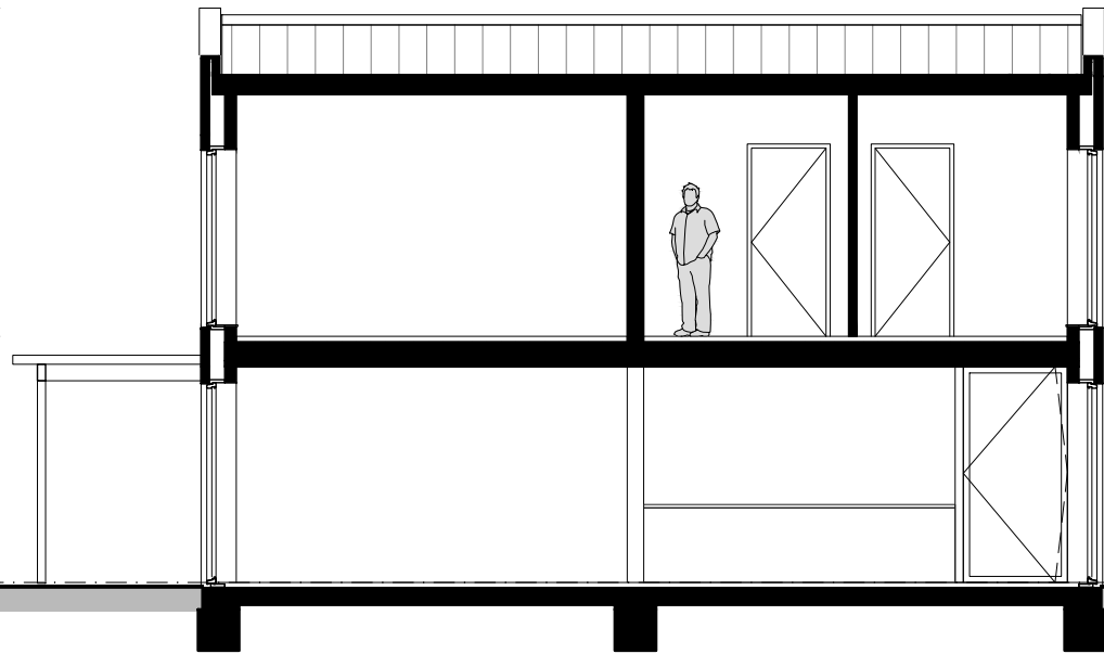
Doorsnede 1
