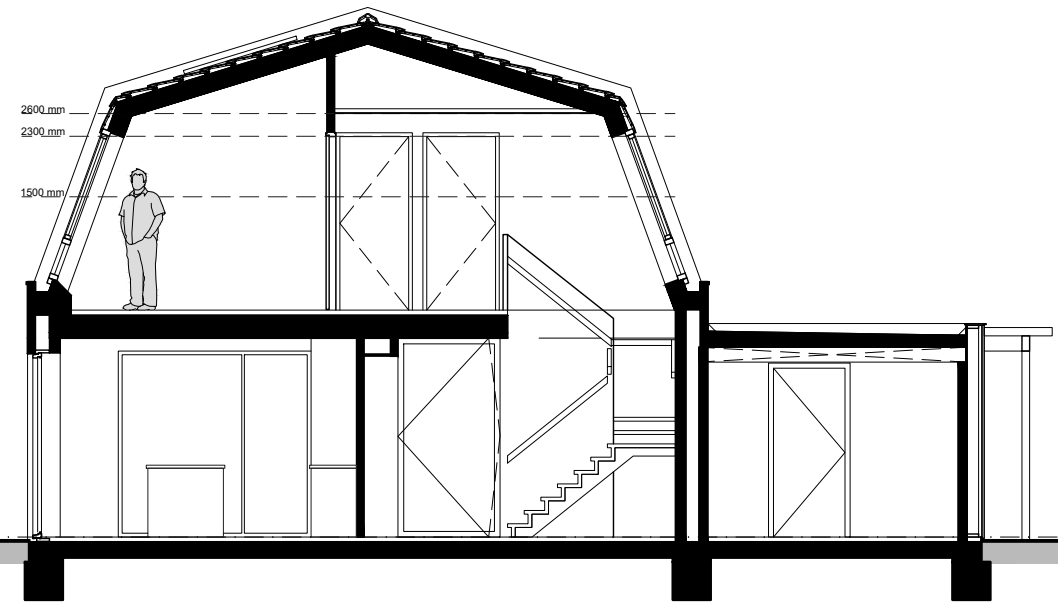
Doorsnede 2
