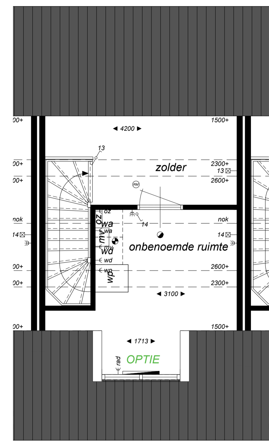
Zolder schaal 1:50
